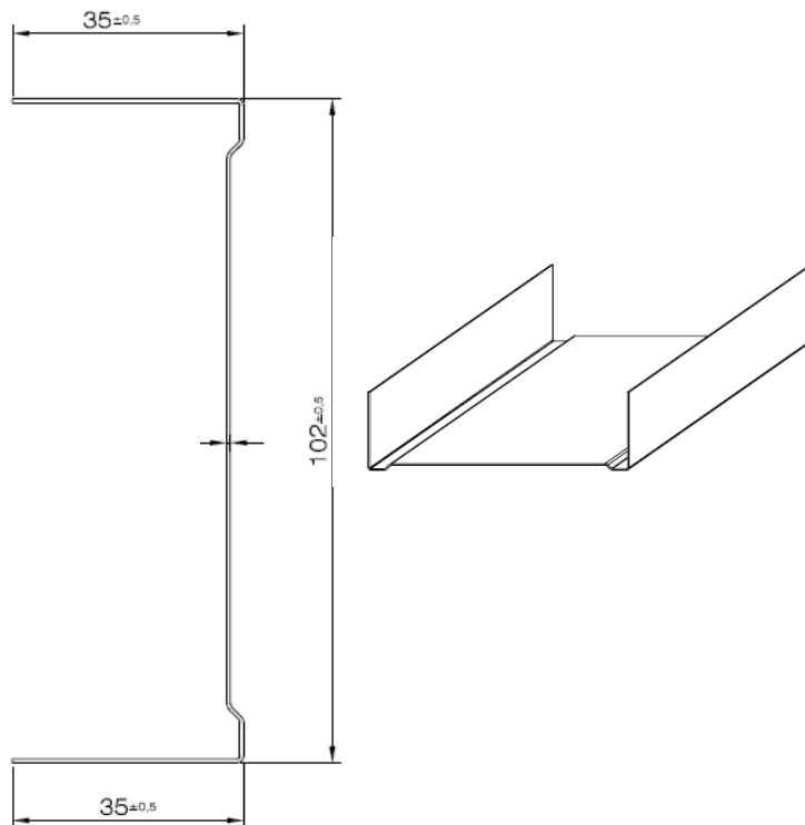
Cotas en mm
