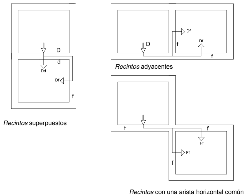
Figura 3.7 Definición de los caminos de transmisión entre dos recintos (Vista en sección vertical).
