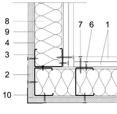
Figura 5.5: Esquina saliente.
