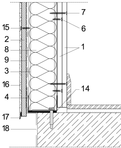
Figura 5.11: Arranque.
