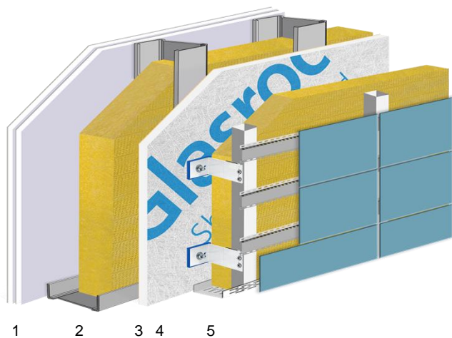
Figura 1.3: Sistema Placotherm® Integra Hoja Simple para su uso como hoja interior de fachada con fachada ventilada (Uso 2).
