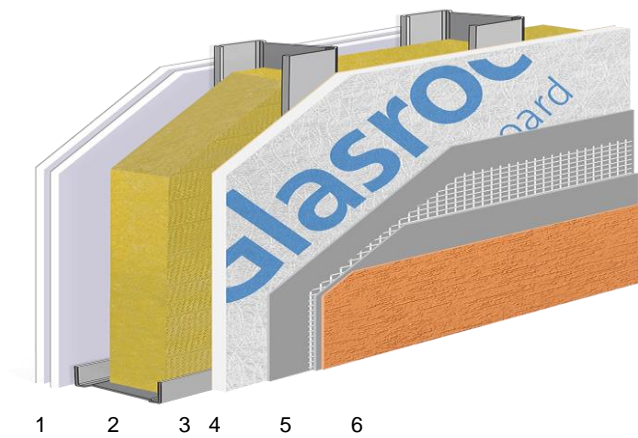
Figura 1.1: Sistema Placotherm® Integra Hoja Simple para su uso como cerramiento completo de fachada (Uso 1).
