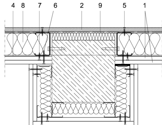
Figura 5.2: Encuentro con pilar.
