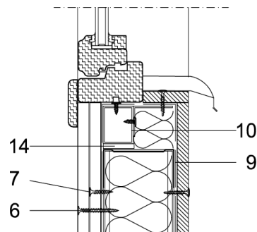
Figura 5.10: Alféizar.
