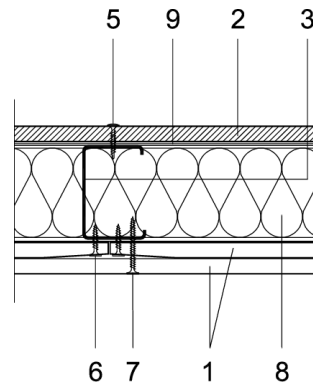
Figura 5.1: Sección horizontal.
