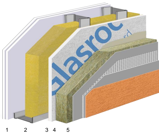
Figura 1.2: Sistema Placotherm® Integra Hoja Simple para su uso como hoja interior de fachada con SATE (Uso 2).
