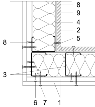
Figura 5.6: Esquina entrante.
