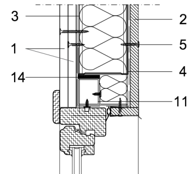
Figura 5.9: Dintel.
