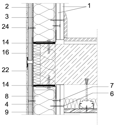
Figura 5.3: Junta de control.
