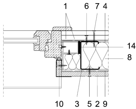
Figura 5.7: Jamba.
