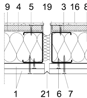
Figura 5.4: Junta vertical de dilatación.
