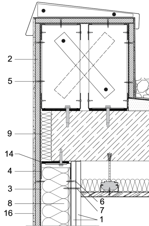
Figura 5.12: Coronación.
