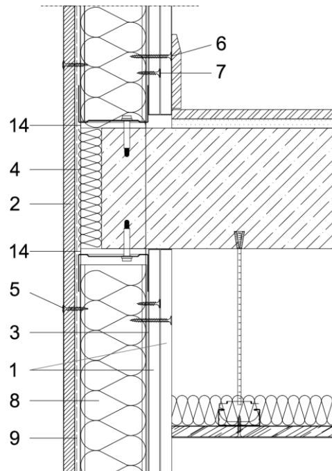
Figura 5.8: Encuentro con forjado.
