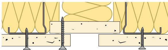
Ejemplo de junta con placa de yeso.
