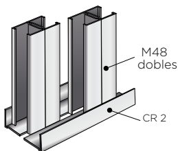
Tabique SAA con angular perfil CR 2
