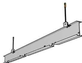
Fijación de la Suspensión Stil Prim® 100 1/4 de vuelta al ala del perfil mediante 2 tornillos TTPF.
