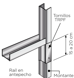
DETALLE B (sin refuerzo)
