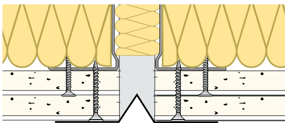
Ejemplo de junta con pieza específica.
