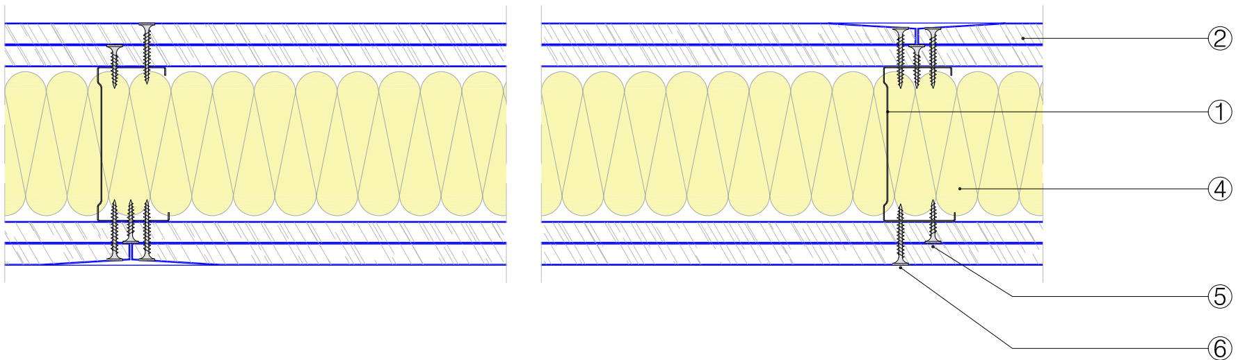
SECCIÓN HORIZONTAL, SISTEMA DE TABIQUE PLACO® 130/90.
