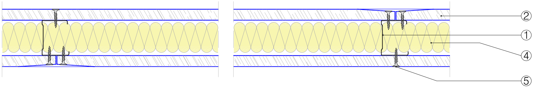
SECCIÓN HORIZONTAL, SISTEMA DE TABIQUE PLACO® 78/48.
