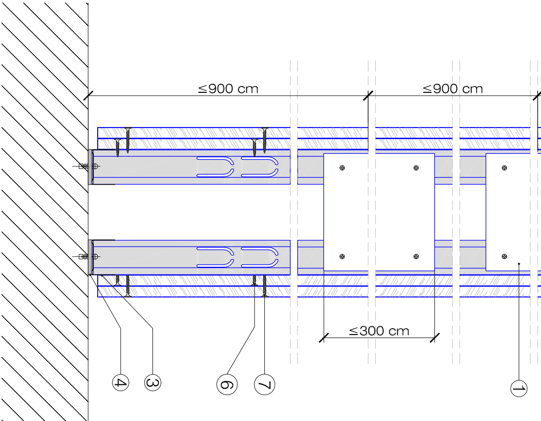
ESTRUCTURA DOBLE ARRIOSTRADA
