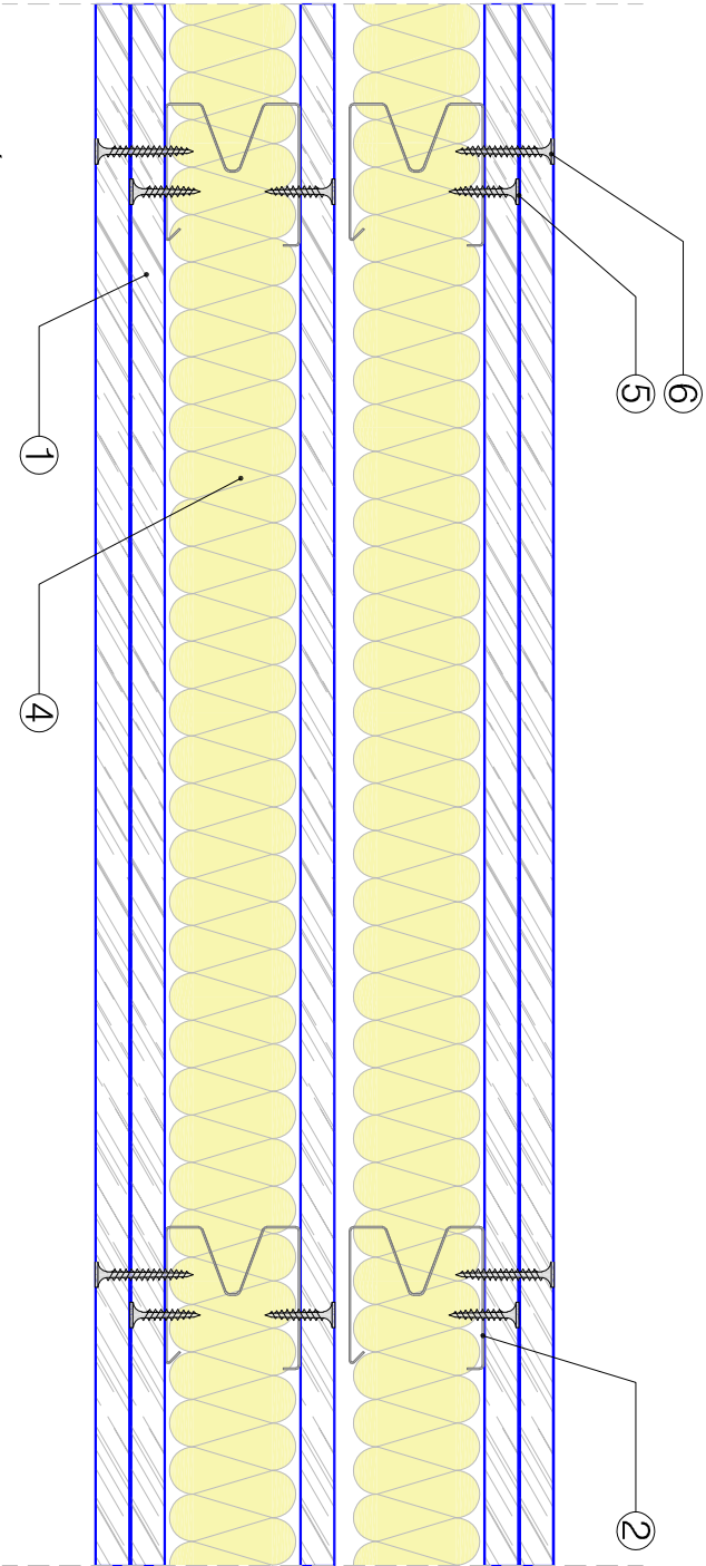
SECCIÓN HORIZONTAL. Escala: 1/3
