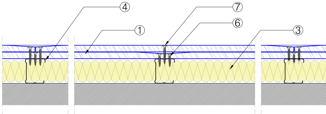
SECCIÓN HORIZONTAL, TRASDOSADO AUTOPORTANTE 73/48
