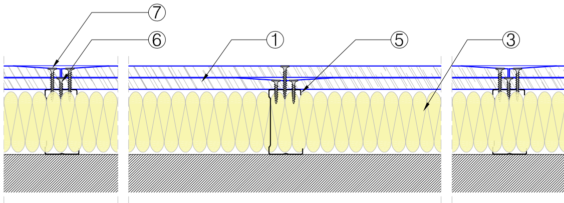
SECCIÓN HORIZONTAL, TRASDOSADO AUTOPORTANTE 95/70
