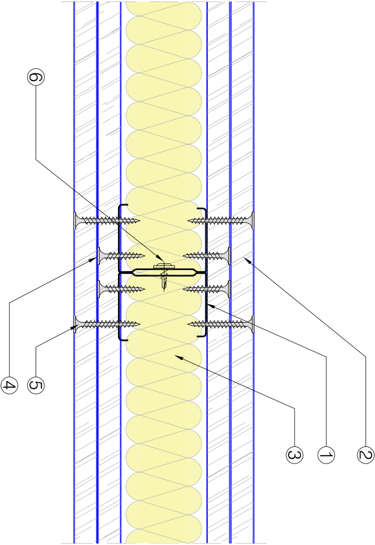
SECCIÓN HORIZONTAL, TABIQUE CON ESTRUCTURA REFORZADA ``H``.
