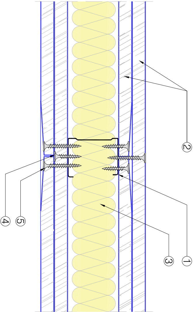
SECCIÓN HORIZONTAL, TABIQUE CON ESTRUCTURA SIMPLE.
