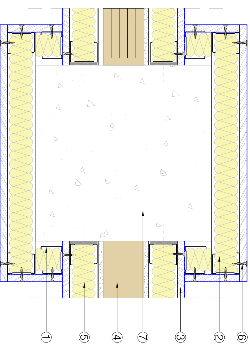
SECCIÓN HORIZONTAL. Pilar de 30x 30 cm.
