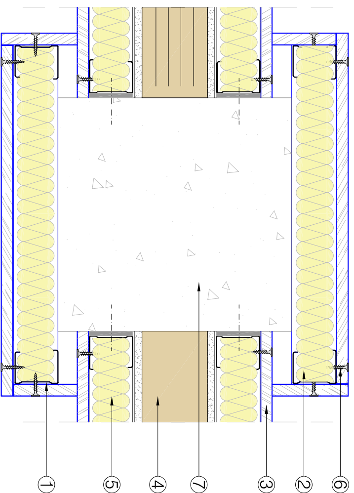
SECCIÓN HORIZONTAL. Pilar de 25x 25 cm.
