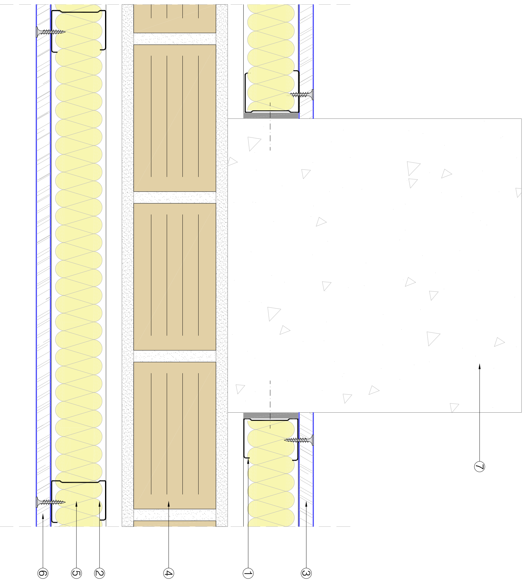
SECCIÓN HORIZONTAL.
