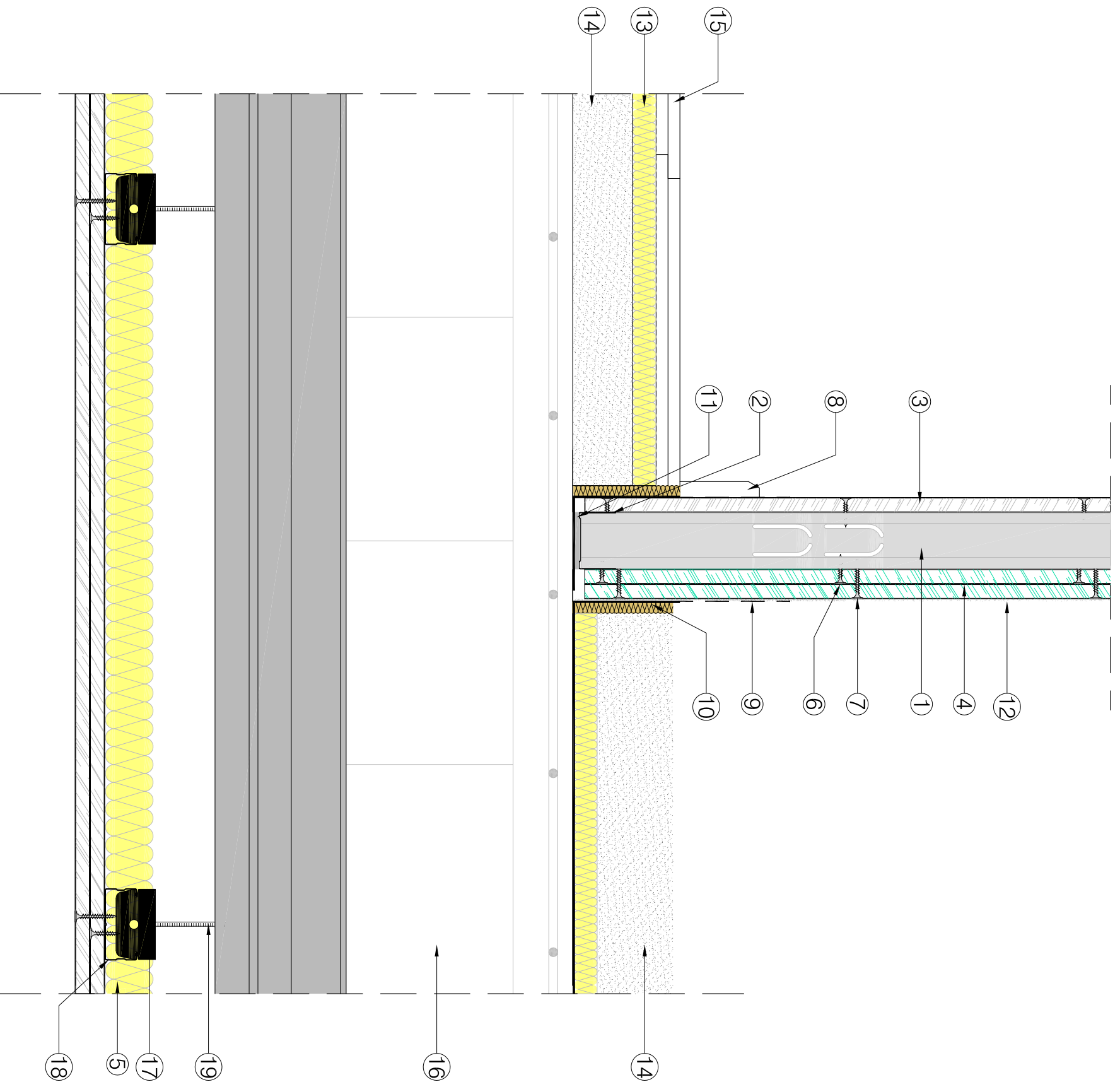
SECCIÓN VERTICAL.
