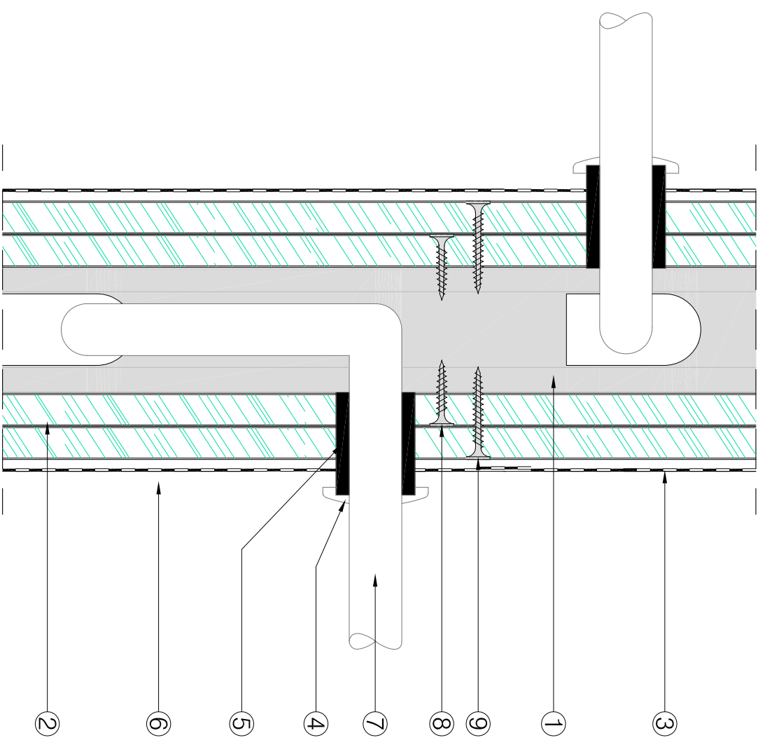
SECCIÓN VERTICAL.
