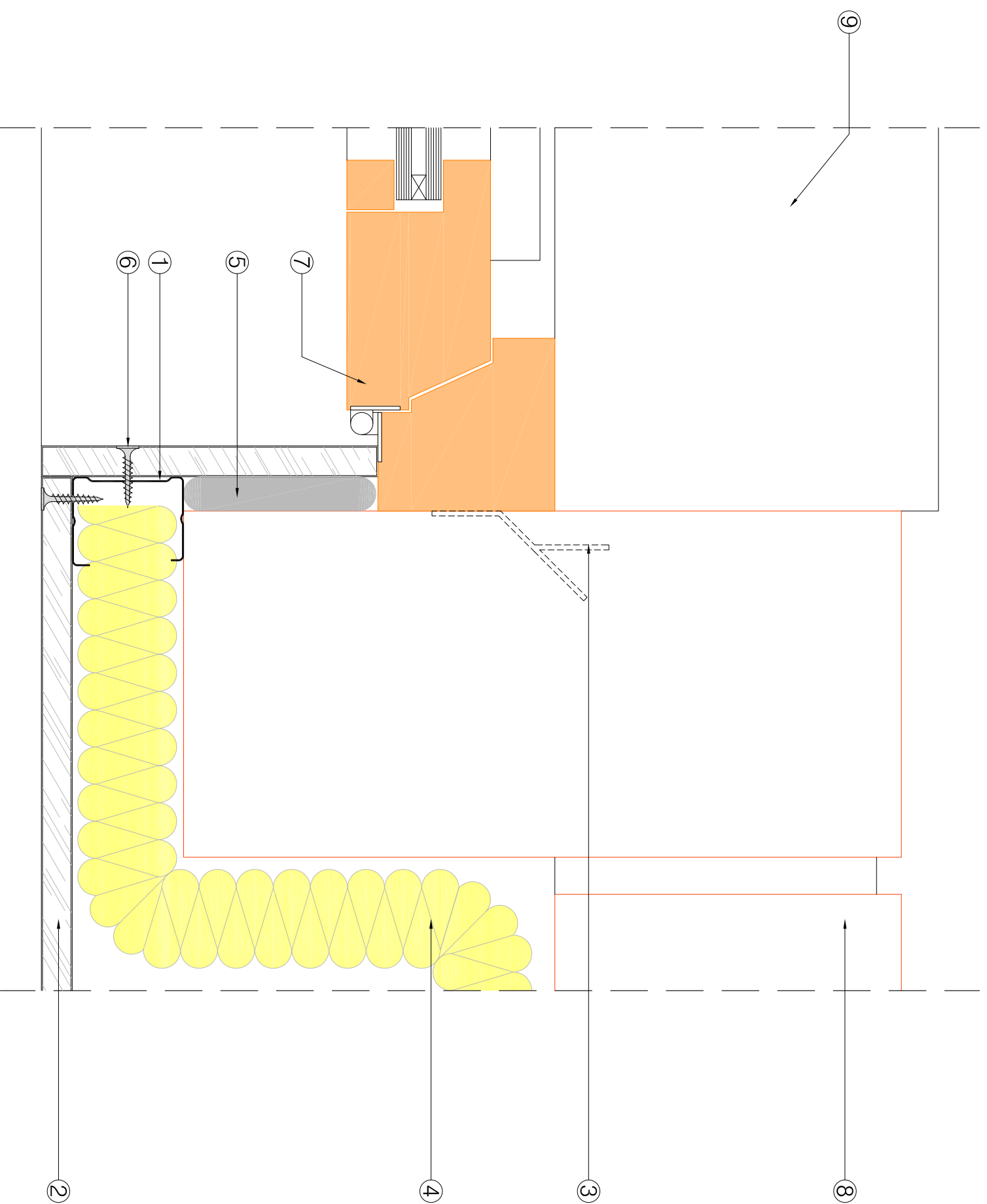
SECCIÓN HORIZONTAL.
