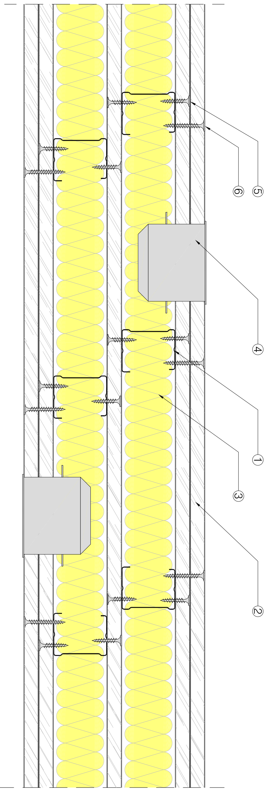
SECCIÓN HORIZONTAL.
