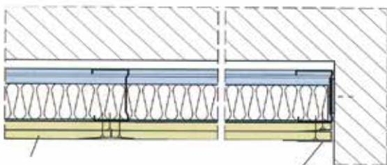
Placa PYL 12,5 mm Tratamiento de juntas
